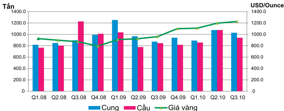
Hình 2. Giá vàng thế giới
